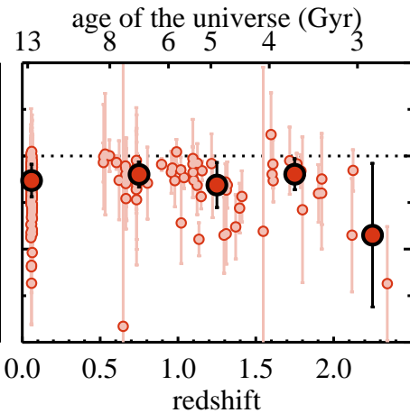
Quiescent
